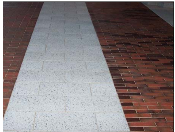
Abb. Nr. 3: Bodenbelag: Das zukünftige Bild der Lingener Fußgängerzone wird geprägt durch Granitstein (in den sog. „Möblierungsbändern“) und dem für Lingen typischen Klinker. Der Klinker wird in seiner Qualität „geschält“, damit ist er auch bei nassen Verhältnissen griffig.
